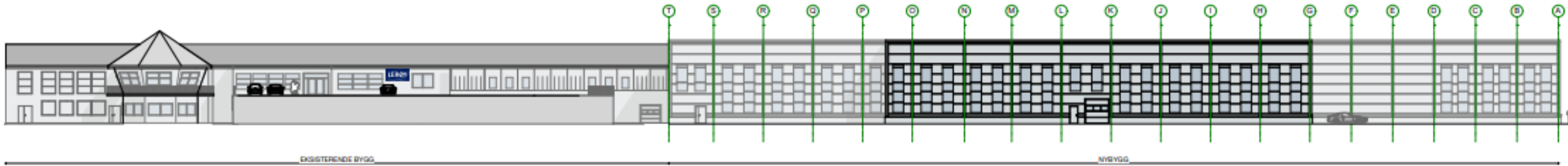
FASADE NORD
